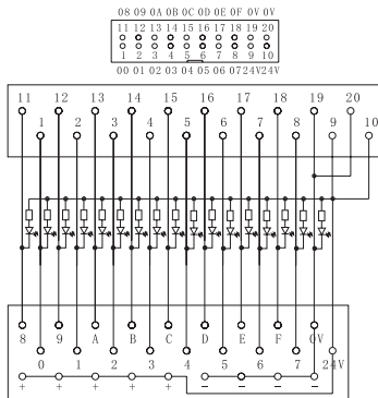
D1012C
