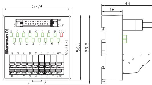
D1012A/D1012A-P
