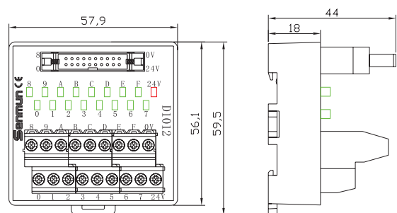
D1012/D1012-P
