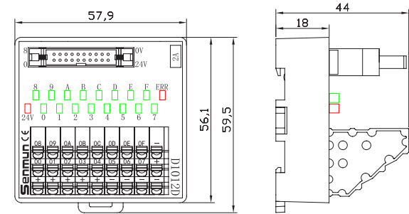
D1012D/D1012D-P
