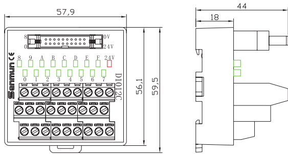
D1012C/D1012C-P
